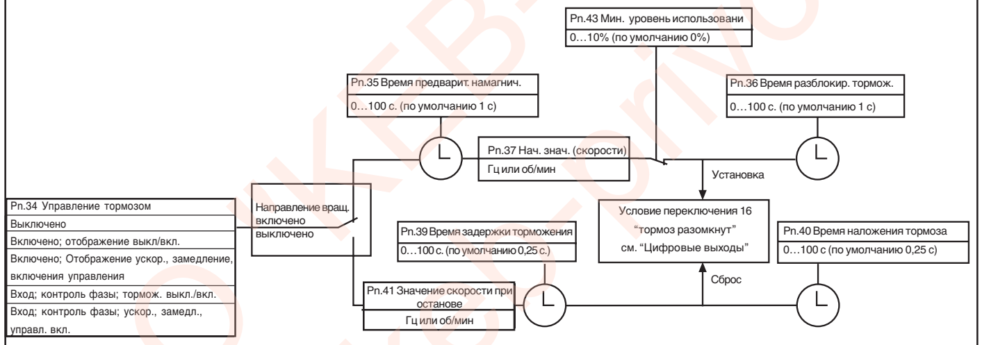
Рисунок 6.9.5.6 Структурная схема функции управления тормозом
