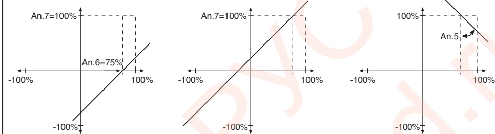
Рисунок 6.2.7.в Смещение X (An.6)=75%; Смещение Y (An.7)= 100%; Коэф. усиления (An.5)= -1.00
