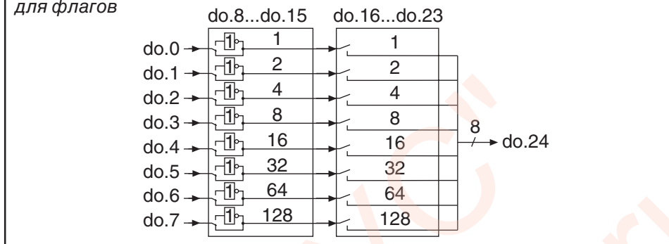
Рисунок 6.3.15 Инвертирование и выбор условий коммутации для флагов
