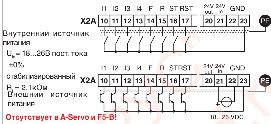
Рисунок 6.3.2.6 Подключение цифровых входов с логикой NPN ( di.0 = 1 )
