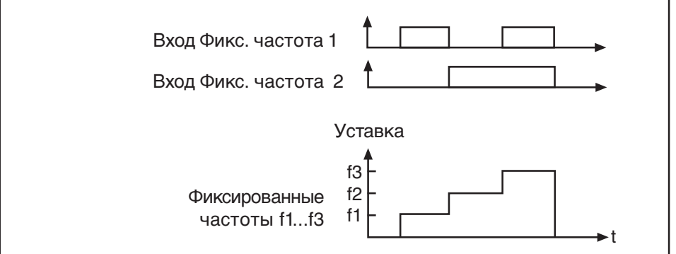
Рисунок 6.4.4.а Выбор фиксированных частот
