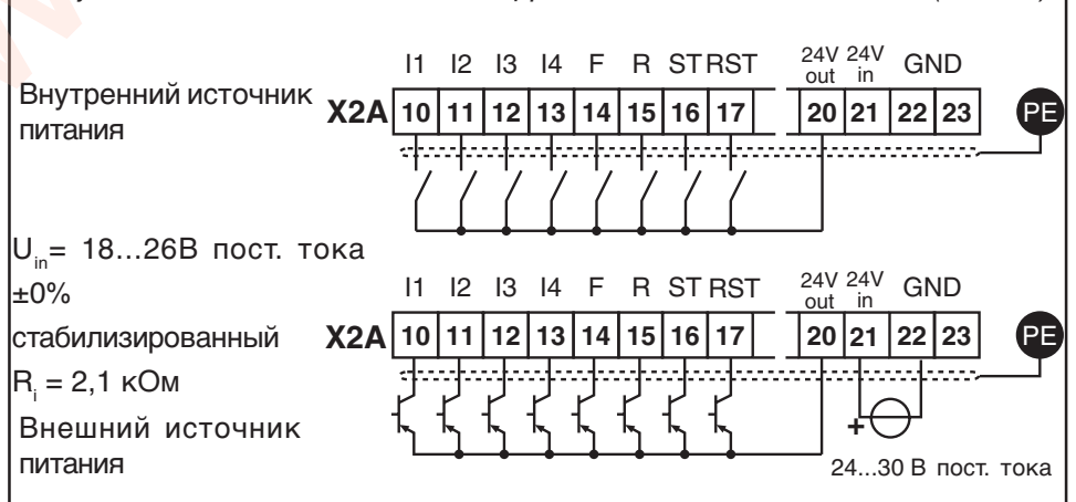
Рисунок 6.3.2.a Подключение цифровых входов с логикой PNP (di.0 = 0)
