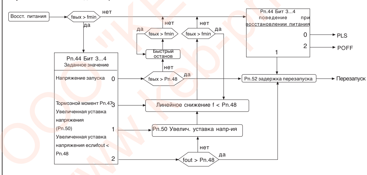
Рисунок 6.9.6.г Поведение при восстановлении питания
