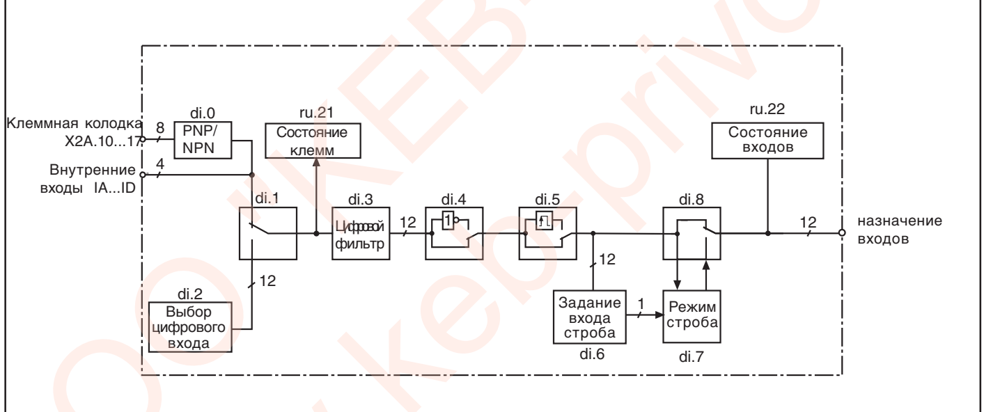
Рисунок 6.3.1 Принципиальная схема цифровых входов
