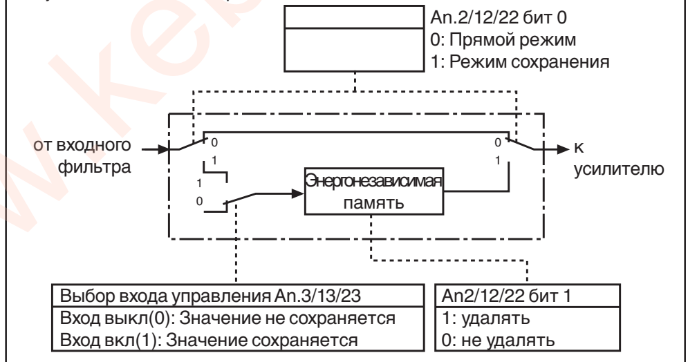
Рисунок 6.2.4 Режим сохранения
