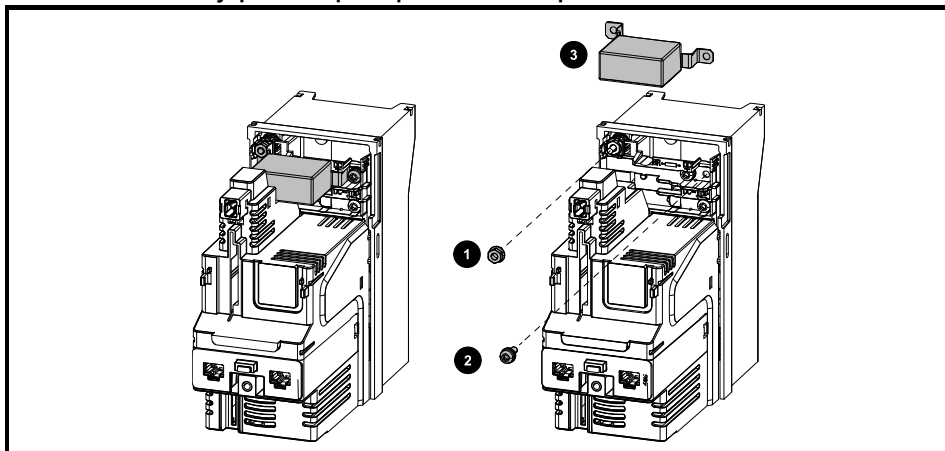
Рис. 3-5 Снятие внутреннего фильтра ЭМС на габарите 3
